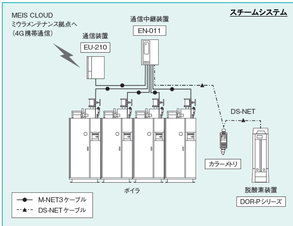
システム構成例 (EU-210の場合)
