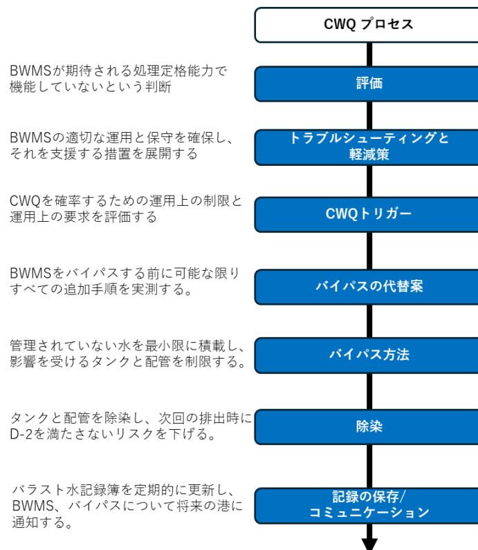
図 CWQ プロセスの概念/概要( MEPC Resolution 387(81)を参照)
