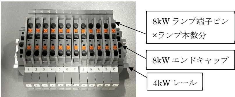
図 3 UV リアクタへ 8kW 用端子台及びエンドキャップの取り付け
