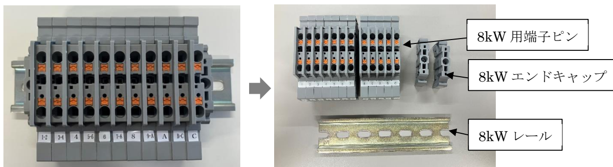
図 5 支給した 8kW 端子台からランプ用端子台及びエンドキャップの取り外し
