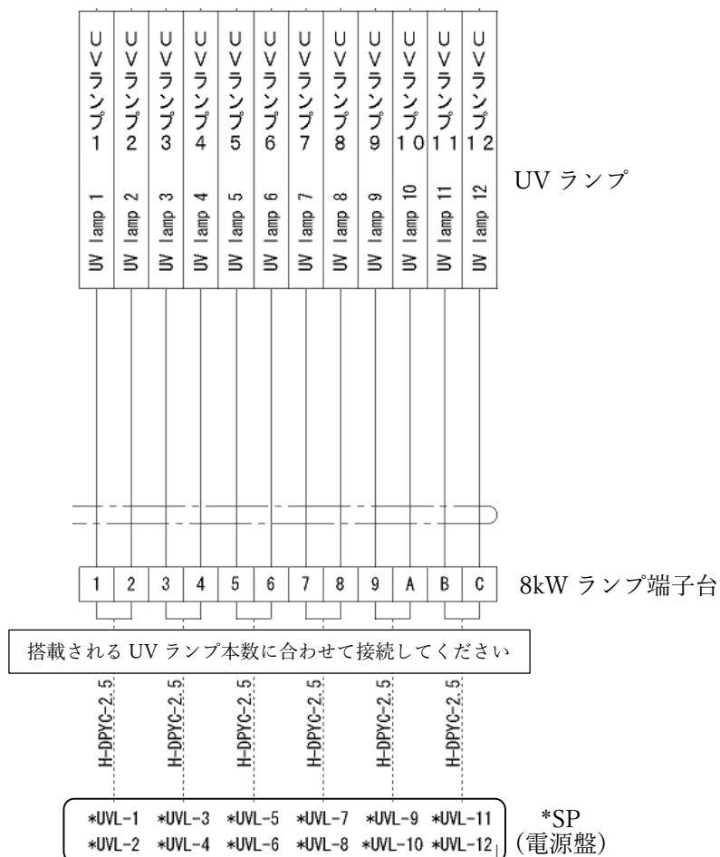
図 7 UV リアクタの配線接続(モータ側)
