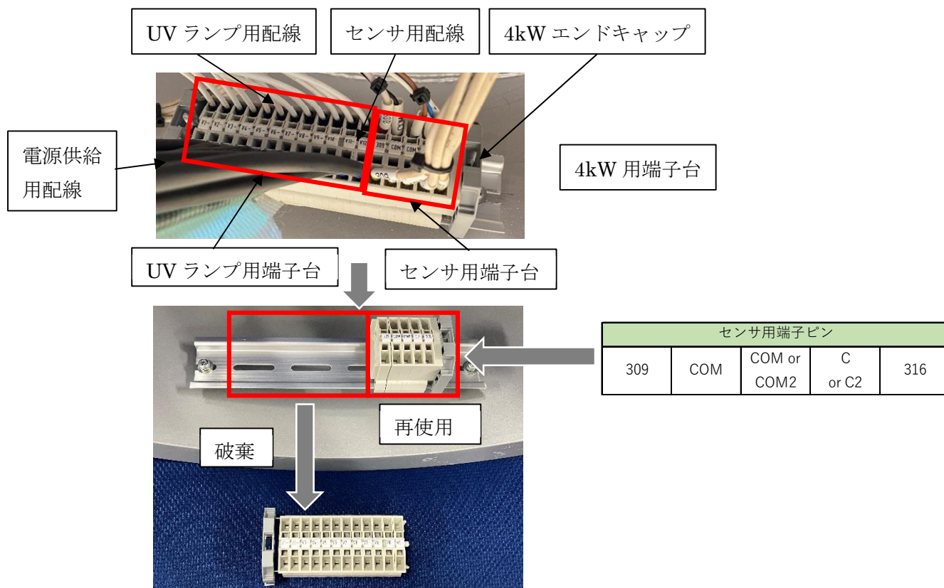
図 4 既設の 4kW ランプ端子台の分解(反モータ側)
