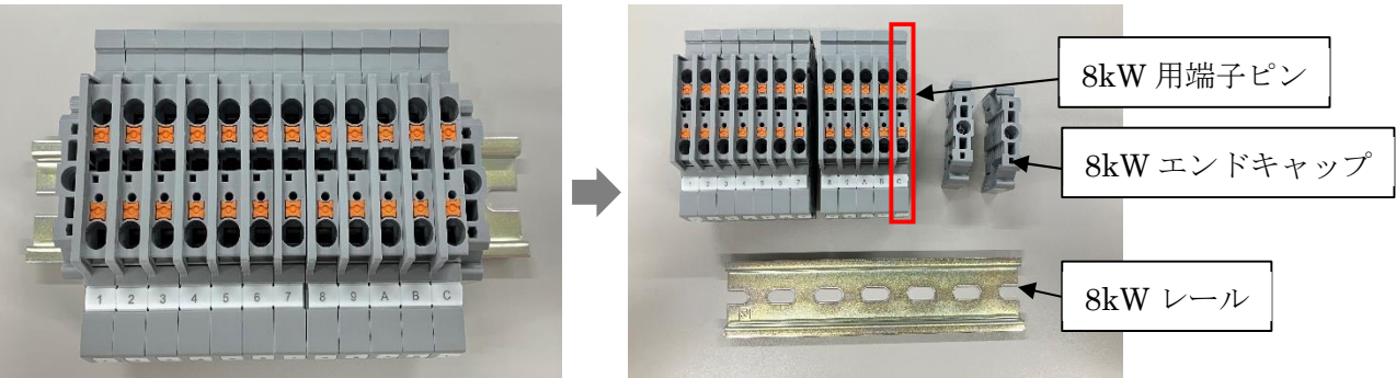
図 2 支給した 8kW 端子台からレールの取り外し
