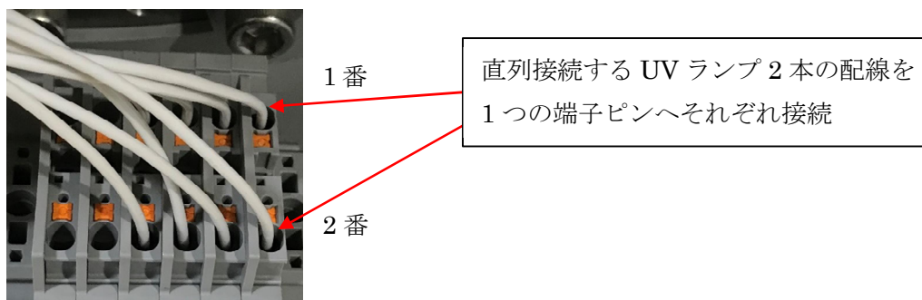
図 8 UV ランプ配線の直列接続（反モータ側）
