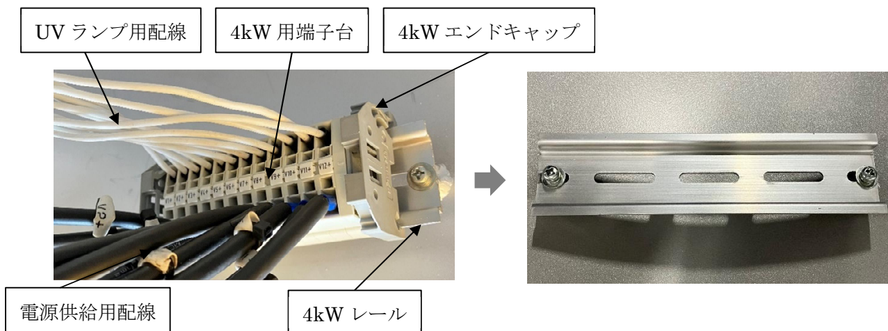
図 1. 既設の 4kW 用端子台の取り外し(モータ側)
